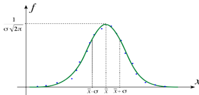
FIGURE – Densité de la loi normale
